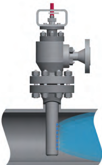
Die Reihenfolge der Öffnung der Düsen ist konstruktiv in der Düsenspindel festgelegt. Die Einspritzung des Kühlwassers beginnt stets mit den in der Mitte des Einspritzkühlers angeordneten Düsen.
